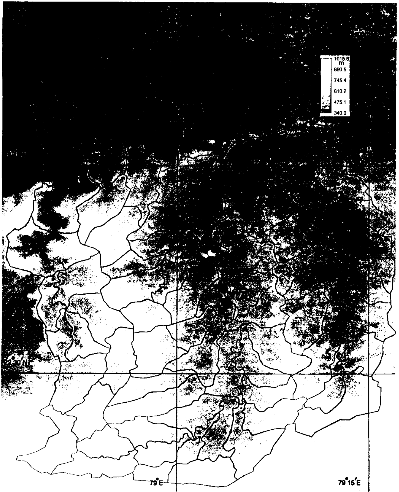
Fig. 5.3 DEM
